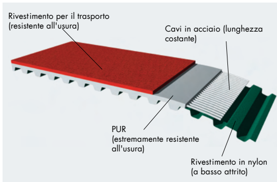
Costruzione della cinghia dentata
