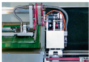
Trasportatore di circuiti stampati
