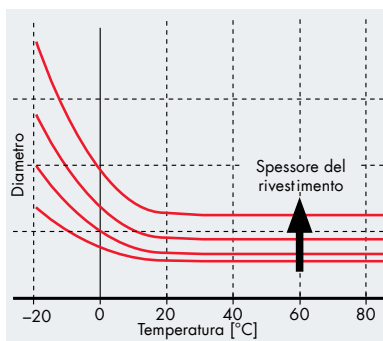
Diametro della puleggia dentata in relazione alla temperatura
