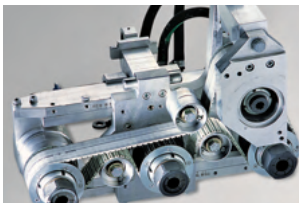
Foratrice a 3 mandrini
