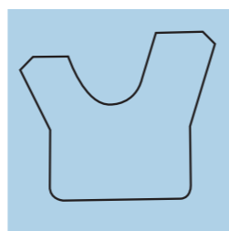
Sezione profilo
